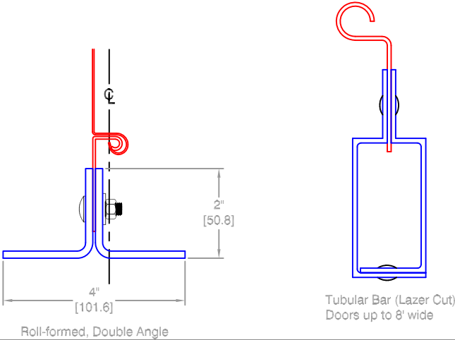
BOTTOM BAR OPTIONS
