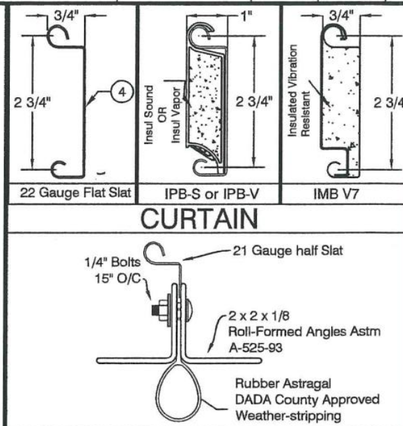
BOTTOM BAR
